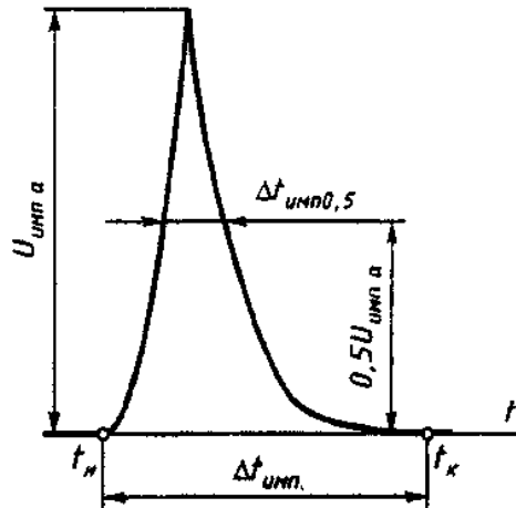
Рисунок Б.3. Параметры импульсного напряжения
