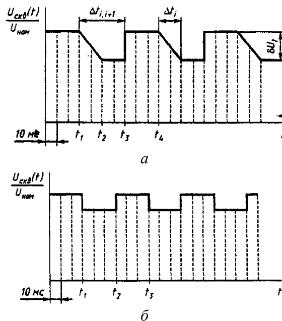
Рисунок Б.1. Колебания напряжения произвольной формы (а) и имеющие форму меандра (б)
